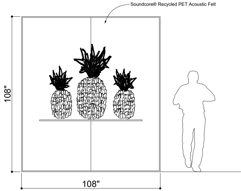
① ELEVATION 1
